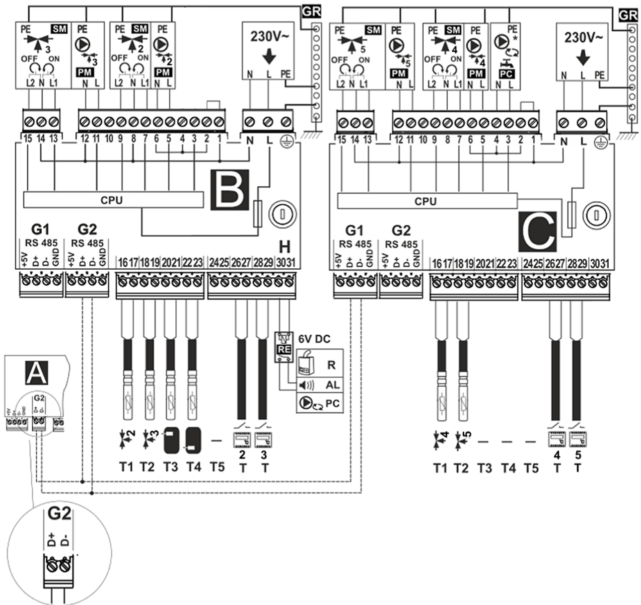
Schemat elektryczny - moduły B i C: T1, T2 – czujnik temp. mieszacza typu CT4, T3 – czujnik temp. górny bufora typu CT4, T4 – czujnik temp. dolny bufora typu CT4, H – wyjście do podłączenia przekaźnika, RE – przekaźnik (6V, max 80mA) do podłączenia kotła rezerwowego R lub alarmu AL, T – termostat pokojowy mieszacza, B, C – moduł rozszerzający, L, N, PE – zasilanie sieciowe 230V~, PM – pompa mieszacza, SM – siłownik mieszacza, PC – pompa cyrkulacyjna, GR – listwa zerowa.
