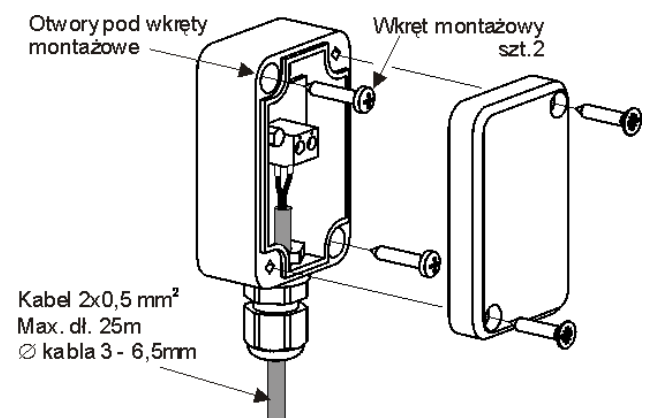
Podłączenie czujnika pogodowego CT6-P.
