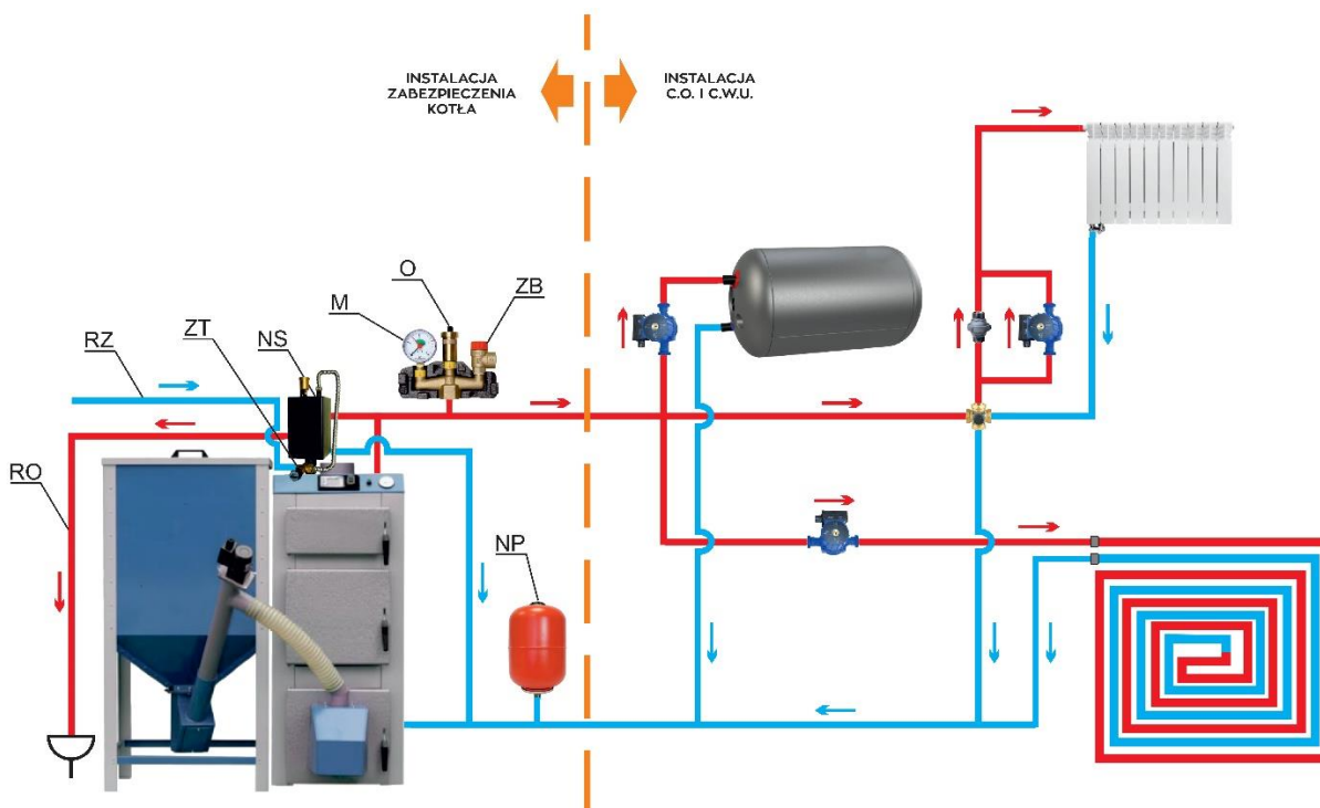
Rys. UZ-1. Schemat montażu kotła typu: PELLPAL® z zewnętrznym systemem schładzającym (naczyniem) przystosowanego do zabezpieczenia w układzie zamkniętym z naczyniem przeponowym.
